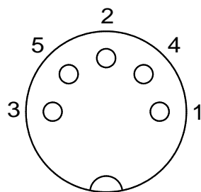
5pol / 180°
